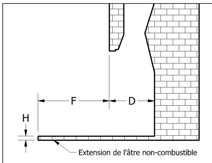
Illustration 3-2 : Dimension minimales requises – vue de côté
