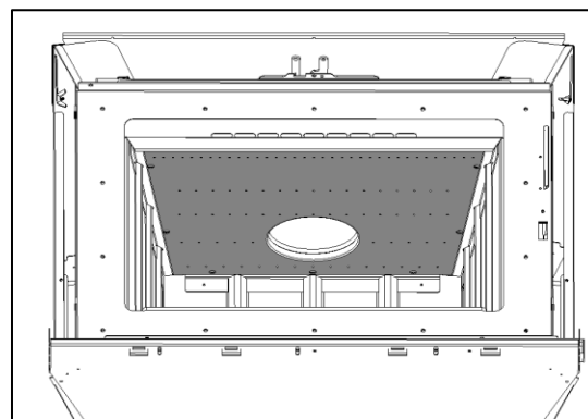
Illustration 2-2: Déflecteur de combustion secondaire à haute performance
