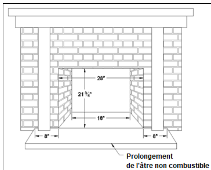
Illustration 11 : Dimensions minimales requises – vue de face
