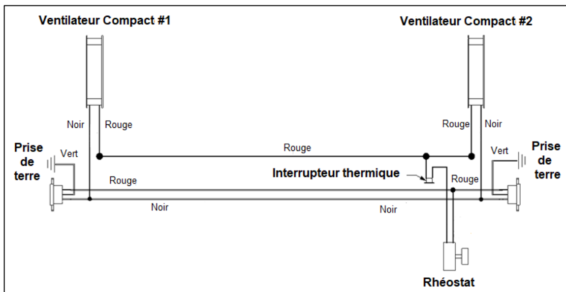
Illustration 19: Branchements électriques
