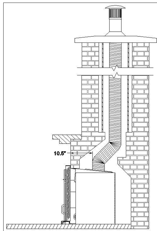
Illustration 17 : Installation du FUSION 18
