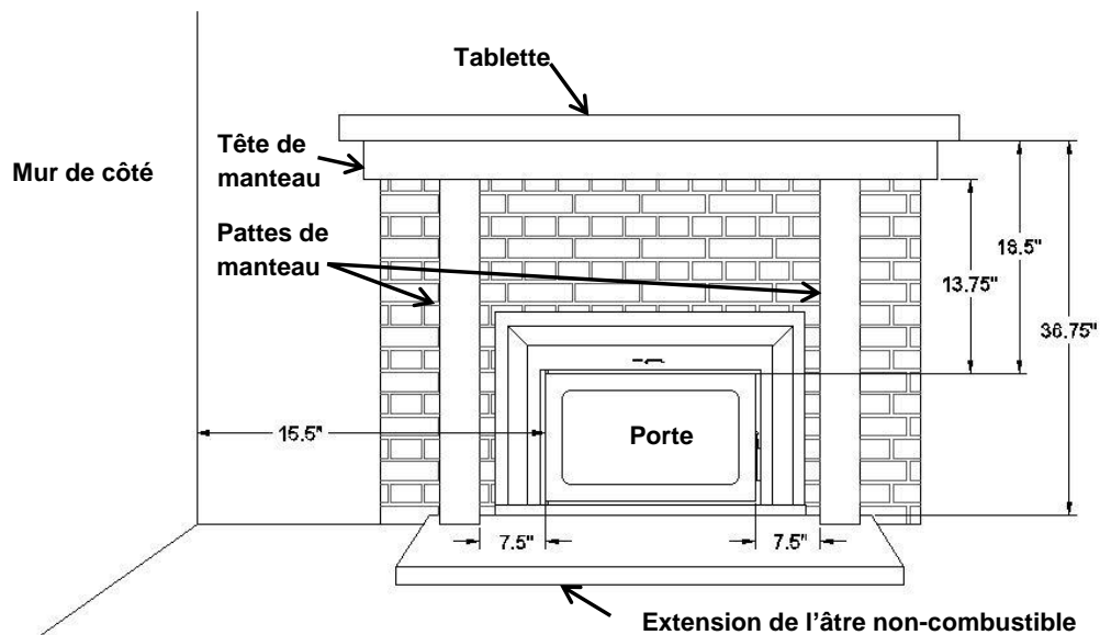
Illustration 20 : Dégagements aux combustibles
