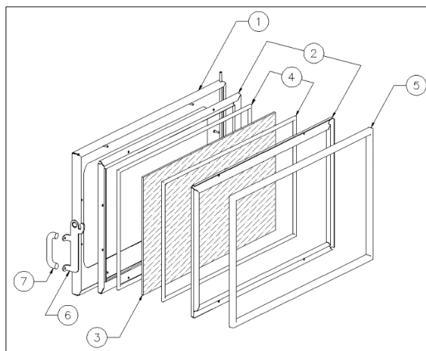
Illustration 24: Remplacement de la vitre
