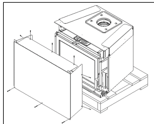
Illustration 13 : Déballage du devant de la caisse
