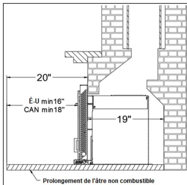
Illustration 12 : Dimensions minimales requises – vue de côté
