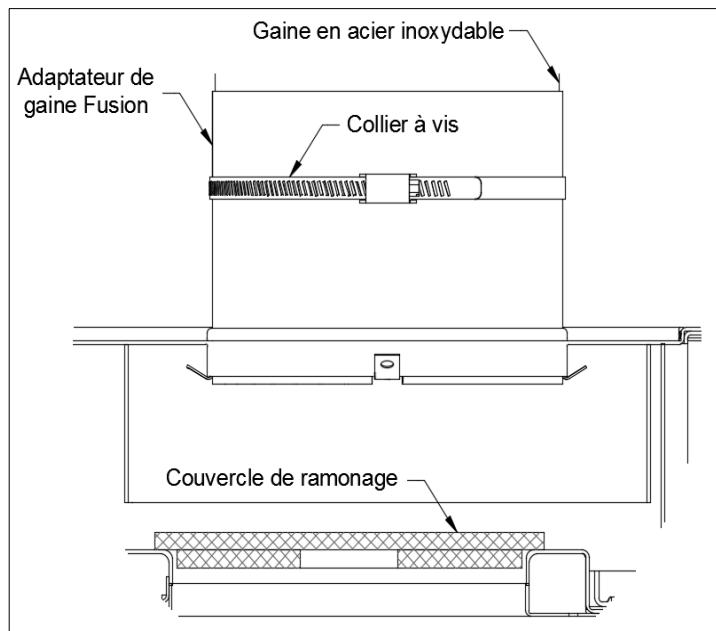
Illustration 15 : Connexion de l'adaptateur et de gaine
