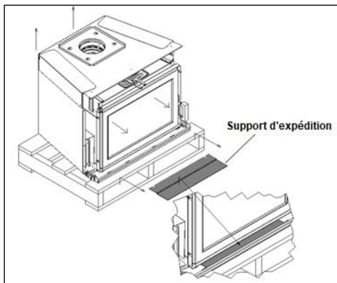
Illustration 14 : Assemblage de la chambre de circulation
