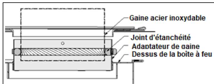
Illustration 16 : Connexion de l'adaptateur et de gaine
