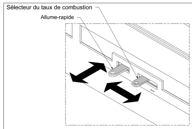
Illustration 3 : Contrôle d'air de combustion
