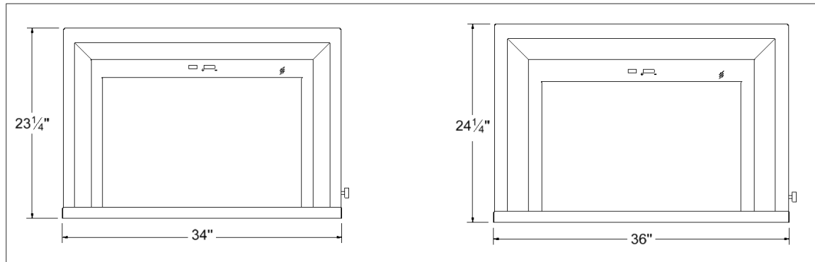
Illustration 6 : Dimensions des deux façades de FUSION 18
