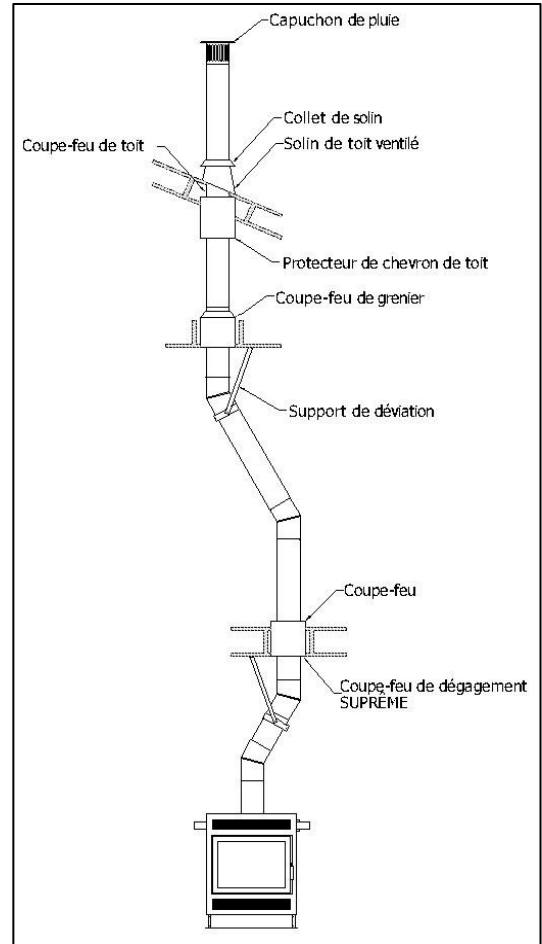
Illustration 3-7 : Installation avec déviation
