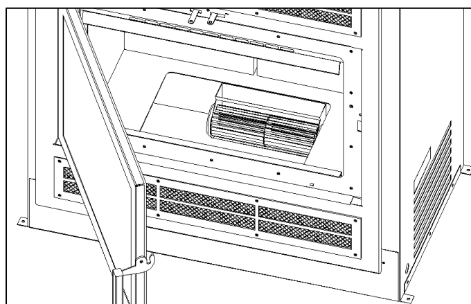
Illustration 3-44 : Accès au ventilateur
