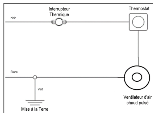
Illustration 4-3: Schéma électrique pour SU250_INL
