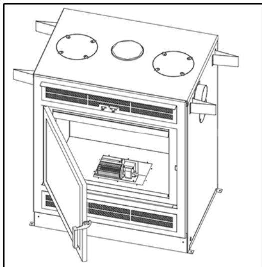
Illustration 3-42 : Accès au ventilateur
