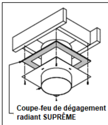
Illustration 2-8 : Coupe-feu de dégagement radiant SUPRÊME
