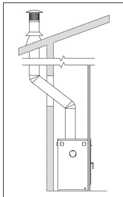
Illustration 3-6 : Installation extérieure
