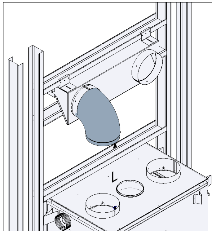
Illustration 3-26 : Coudé installé temporairement sur l'adaptateur linéaire conduit/grille
