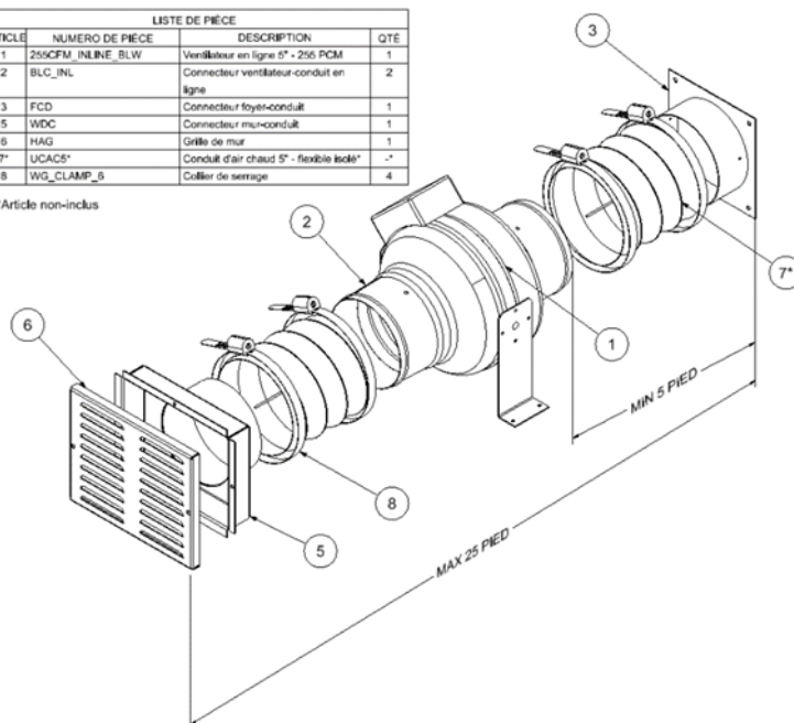
Illustration 4-2: Liste des pièces - SU250
