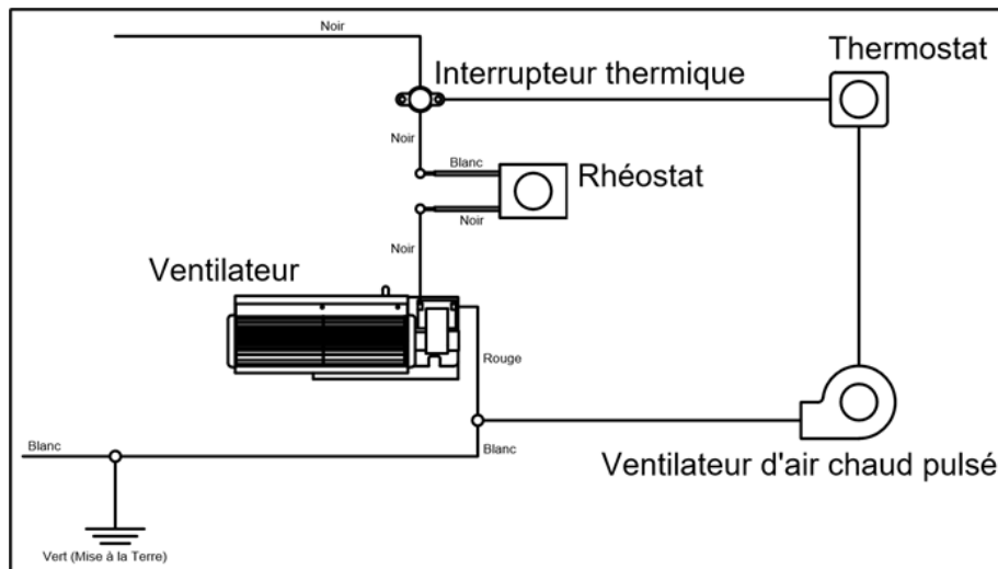
Illustration 4-4: Schéma électrique (connexion en parallèle) pour SU250 et ensemble de ventilateur
