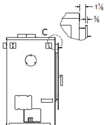
Illustration 2-3 : Dimensions Éléance 42 contemporain rectangulaire
