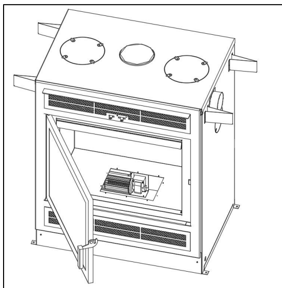
Illustration 3-44 : Accès au ventilateur
