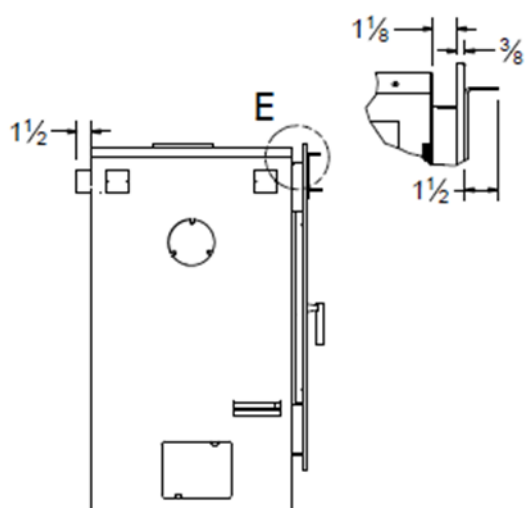
Illustration 2-1 : Dimensions Éléance 42 traditionnel rectangulaire
