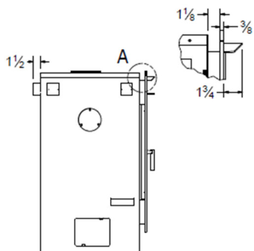
Illustration 2-2 : Dimensions Éléance 42 traditionnel arqué
