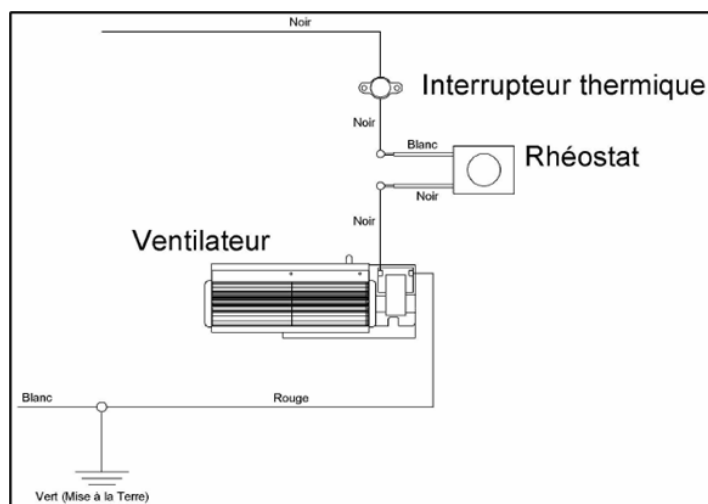
Illustration 3-45 : Diagramme électrique
